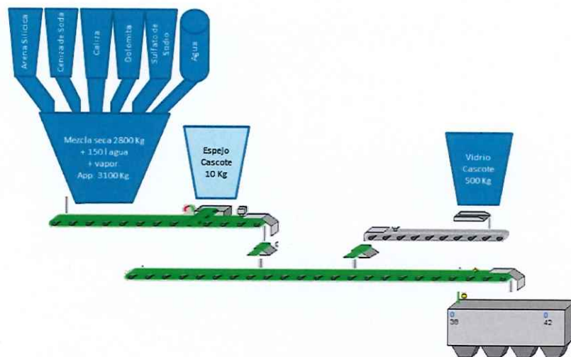
Imagen 1. Diagrama de adición de Materias Primas
